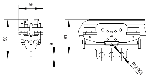
Laufwagen HD / Conducteur HD / HD Runner = HD
