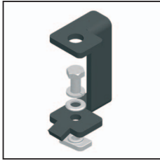
3115 8051 Schienenabhangung für doppelte, obenliegende Seilführung / Entretoise de suspension - double guidage supérieur / Double Top Cord Suspension Bracket
