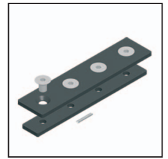
3115 0011 Schienenverbinder (nicht sichtbar) / Raccord de rail (non visible) / Track Splice (not shown)
