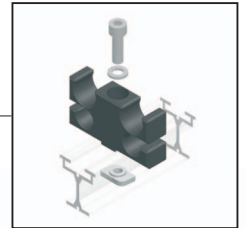
3115 5011 Seilführung, gerade Schiene / Guidage de drisse - section droite / Double Top Cord Guide
