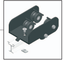
3115 5041 Ableitrolle / Poulie de tirage - vers le bas / Head Pulley, double cord
