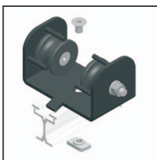
3115 5031 Umlenkrolle / Poulie de renvoi / Return Pulley
